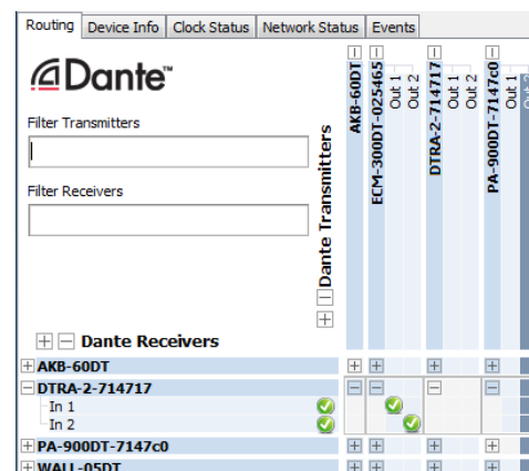
Schéma 4 Routage du ECM-300DT vers le DTRA-2
