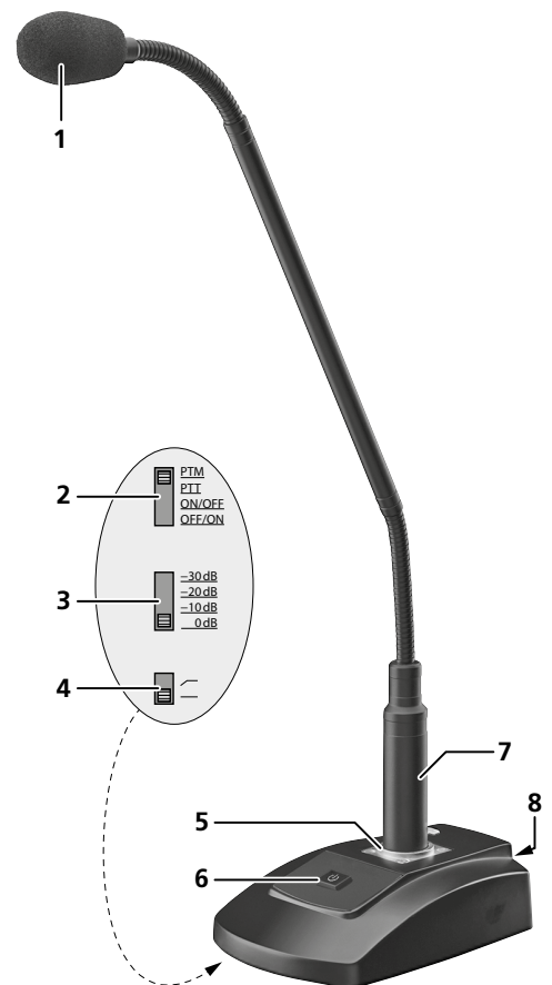
Schéma 2 Eléments de fonctionnement et branchements
