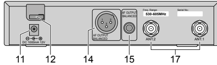
Schéma3 Branchements
